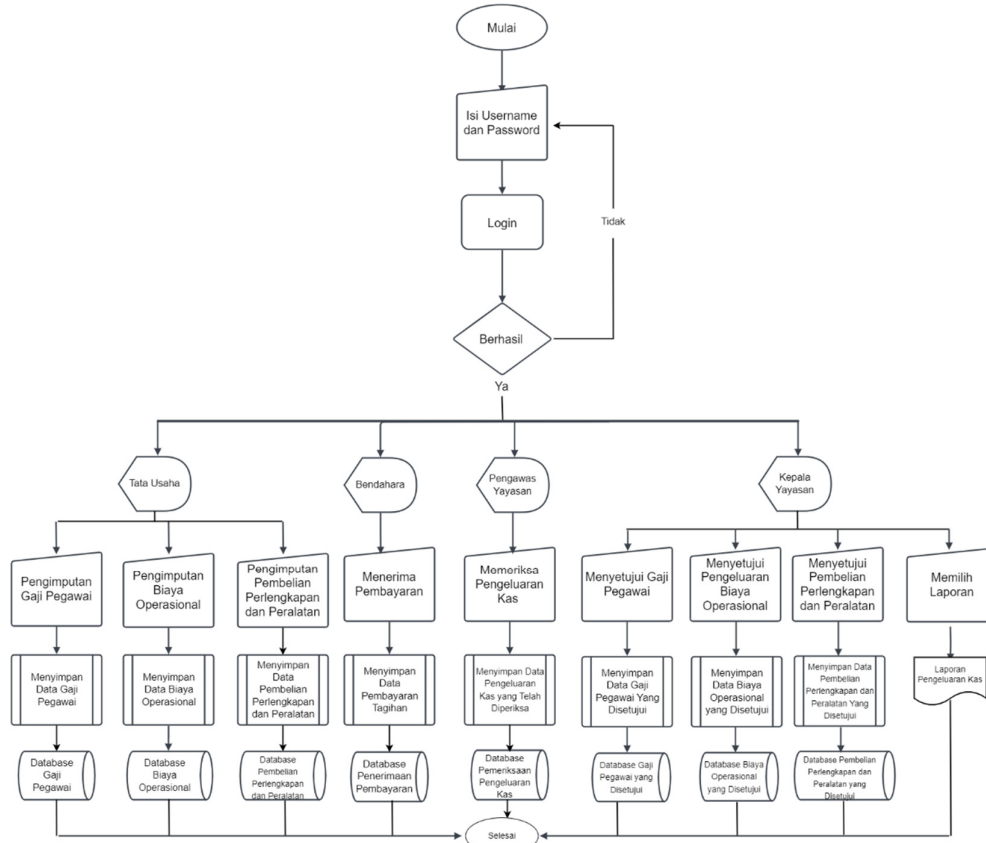
Flowchart Data Master Pengeluaran Kas
