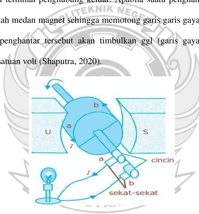
Gambar 2.2 Prinsip Kerja Generator
