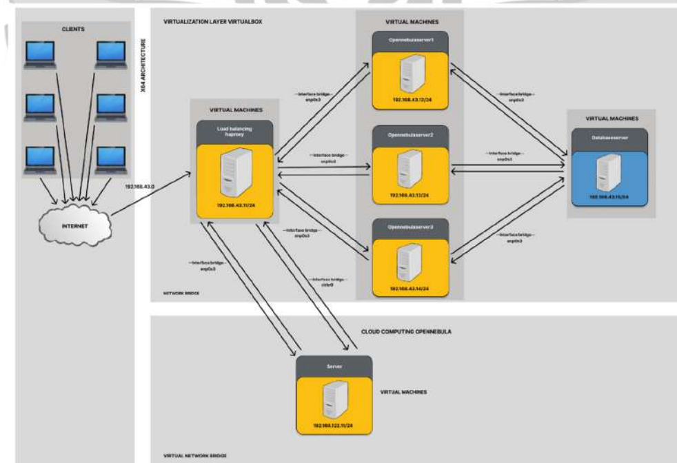
Gambar 3.4 Skema Jaringan
