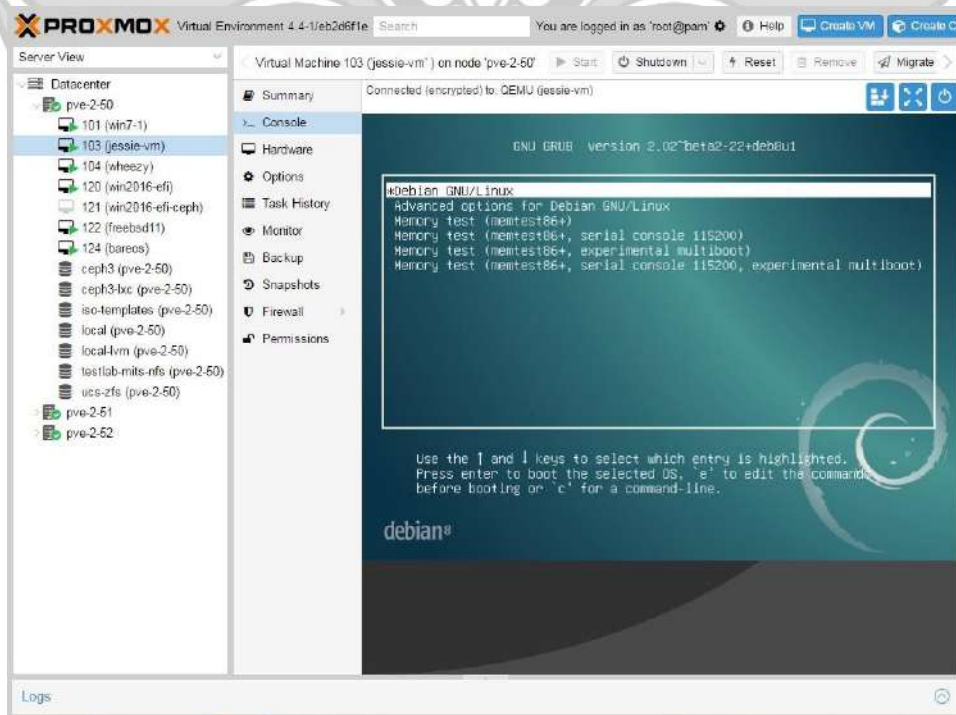
Gambar 2.5 Proxmox VE
