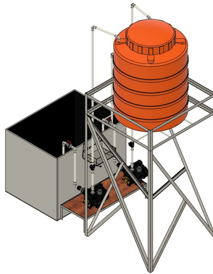
Gambar 1. Desain rancangan struktur kerangka keseluruhan
