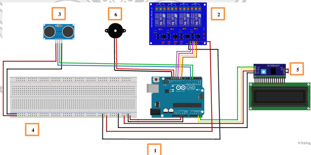
Gambar 2. Skema Rangkaian Sitem
