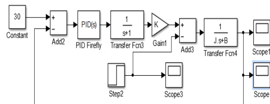
Gambar 11. Pemodelan motor sinkron control PID Firefly
