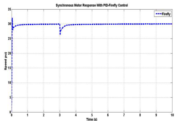
Gambar 12. Respon kecepatan motor sinkron control PID Firefly
