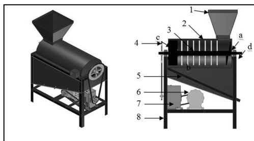
Gambar 4. Konstruksi mesin pemisah bunga cengkeh
