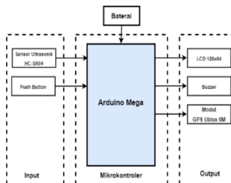
Gambar 5 Diagram Blok Perancangan Sistem Perangkat Keras
