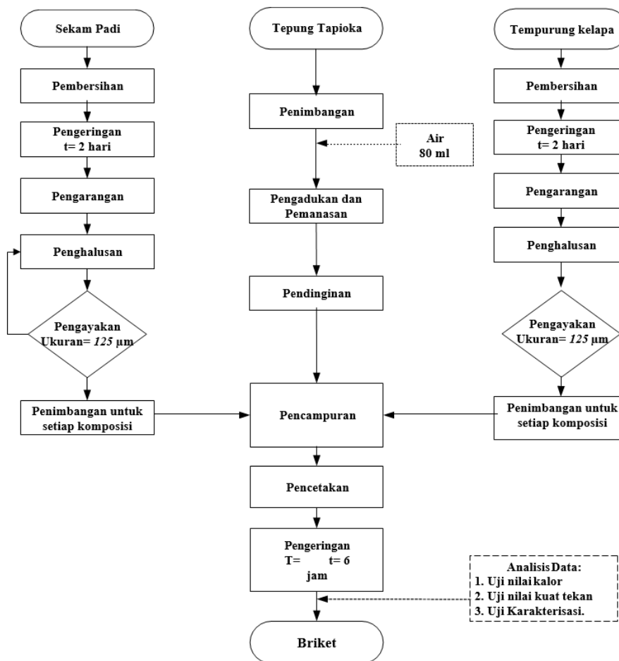
Gambar 1. Diagram Alir Pembuatan Biobriket Campuran Arang Sekam Padi dan Arang Tempurung Kelapa
