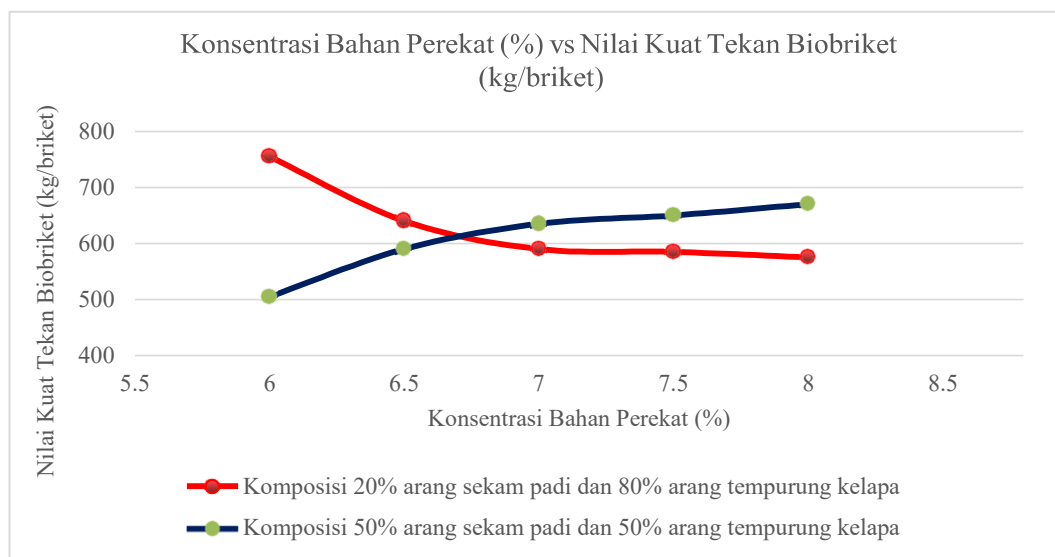
Gambar 3. Hubungan konsentrasia bahan perekat (%) dan nilai kuat tekan biobriket (Kg/briket)
