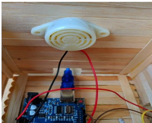
Gambar 4.b. Sistem sensor FR-04 pada Atap Jemuran
