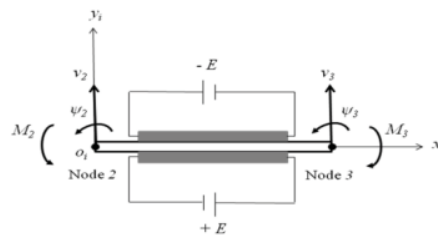
Fig. 6. Modeling piezoelectric actuator
