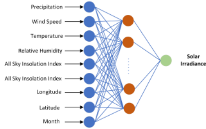
Fig. 2. ANN Layers
