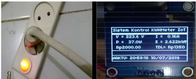
Gambar 10. Pengujian Alat dan Beban
