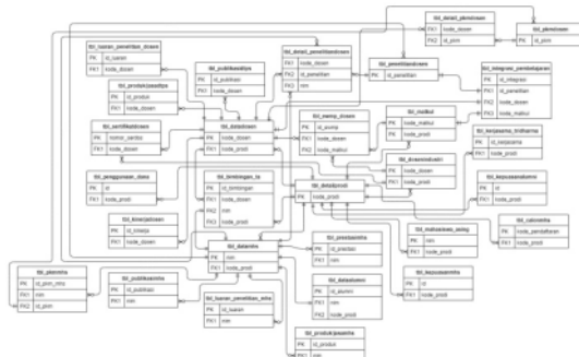
Gambar 8. E-R Diagram Konseptual Sistem Akreditasi PNUP
