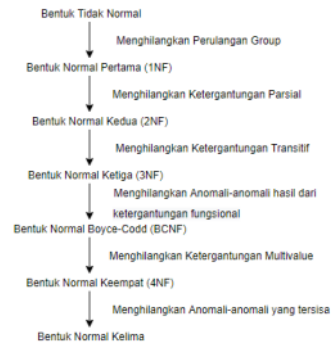
Gambar 3. Bentuk Tahapan Normalisasi
