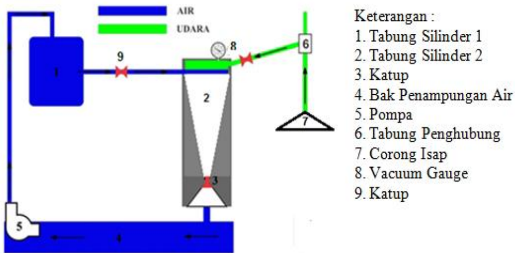
Gambar 2.1. Instalasi Ejektor Hasil Rancang Bangun
