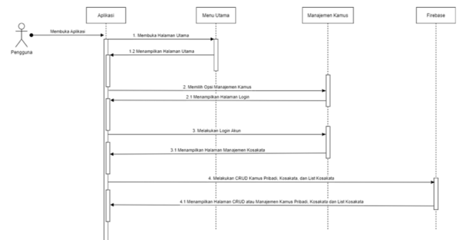
Gambar 5. Sequence Diagram Manajemen Kamus
