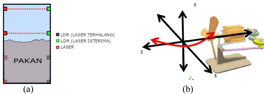
Gambar 3 (a) Pengukuran level pakan dalam tangki dan (b) Ilustrasi mekanisme pelontar pakan
