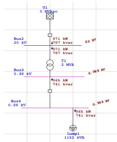
Gambar 6. Hasil simulasi sebelum perbaikan faktor daya
