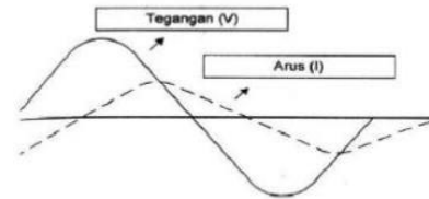
Gambar 1. Faktor Daya Lagging
