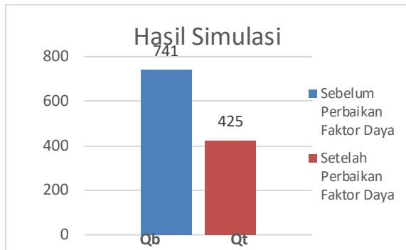
Gambar 8. Perbandingan daya reaktif sebelum dan setelah perbaikan faktor daya
