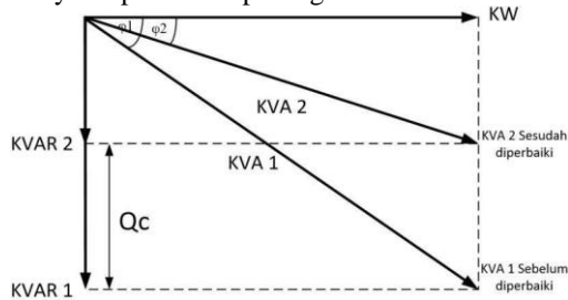
Gambar 3. Diagram daya untuk menentukan daya kapasitor
