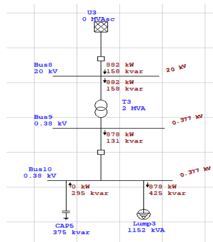
Gambar 7. Hasil simulasi setelah perbaikan faktor daya
