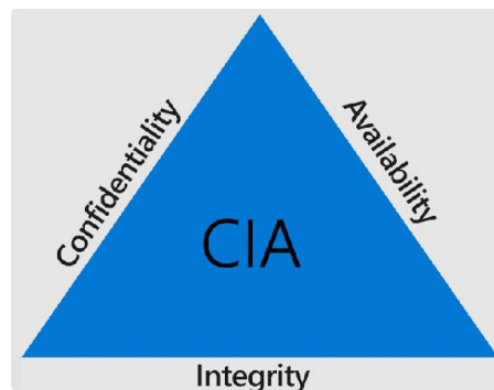
Gambar. 1 CIA Triad
