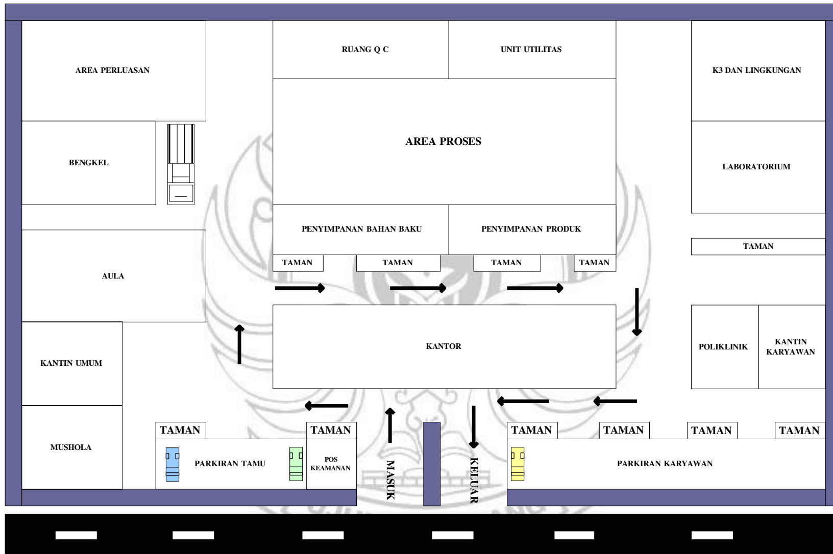
Gambar 9.1 Tata Letak Pabrik
