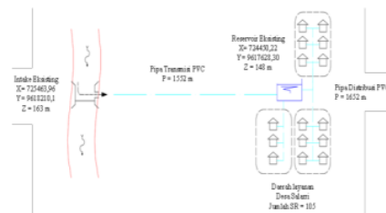
Gambar 3. Skema jaringan eksisting Desa Salarri
