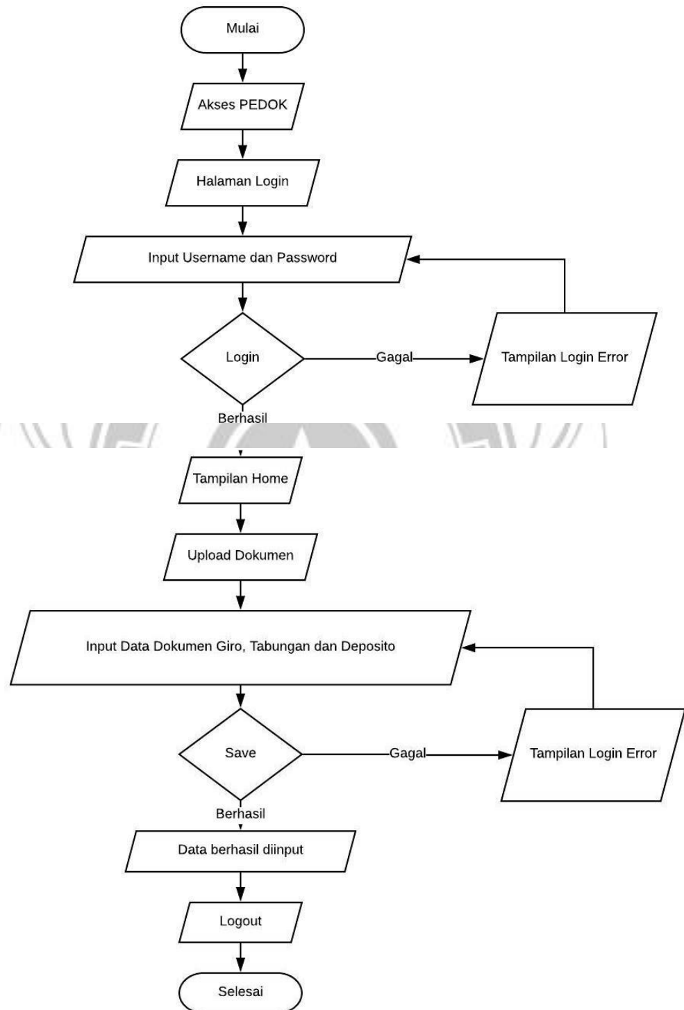
Gambar 3.3 Tampilan Flowchart Pengujian
