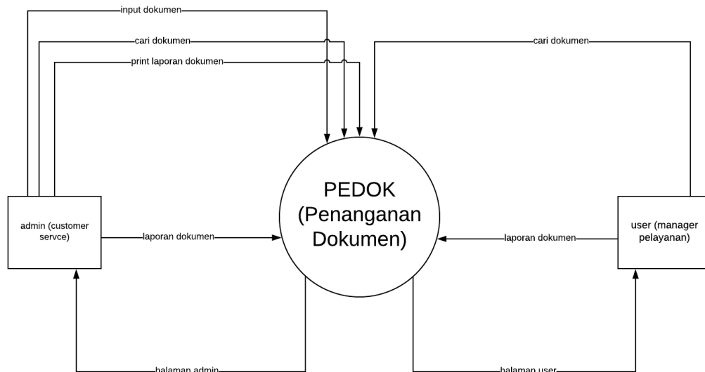
Gambar 3.2 Tampilan Konsep Alir Data
