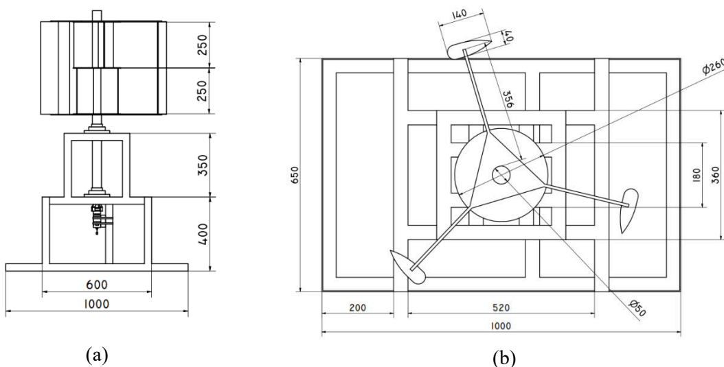
Gambar 1. Dimensi hybrid turbine VAWT (a) tampak depan dan (b) tampak atas
