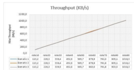
Gambar 11 Grafik throughput dengan menggunakan metode least connection
