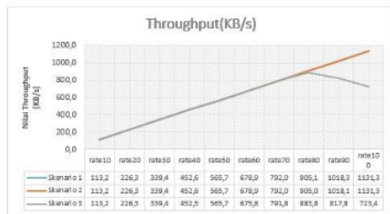
Gambar 10 Grafik throughput dengan menggunakan metode Round robin
