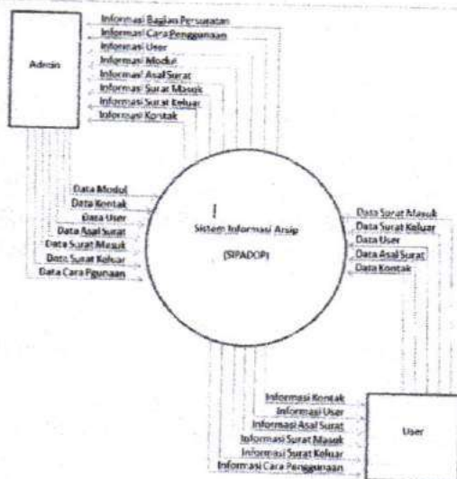
Gambar 1 : Diagram Konteks atau DFD Level 0
