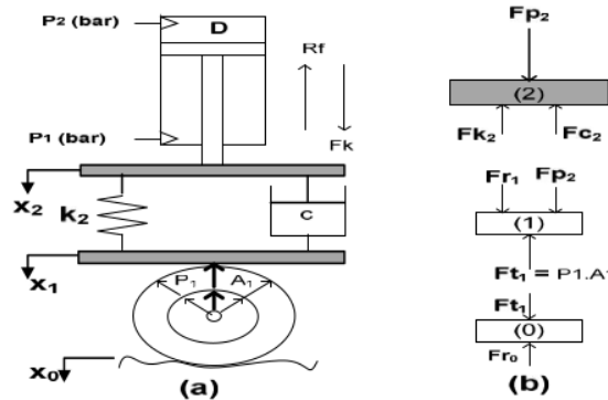
Gambar 2, Mekanisme pembebanan ekperimental sistem pneumatic
