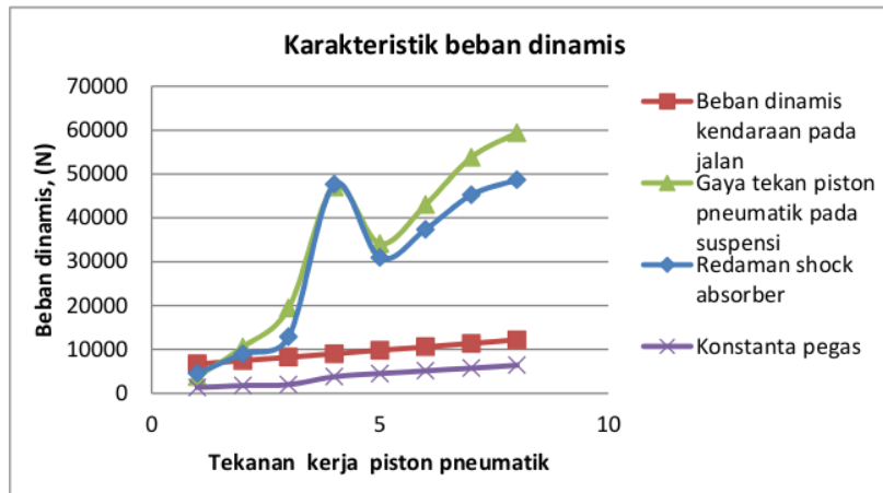
Gambar 5 Karakteristik beban dinamis oleh gaya piston, F_{p2} terhadap pegas dan shock
