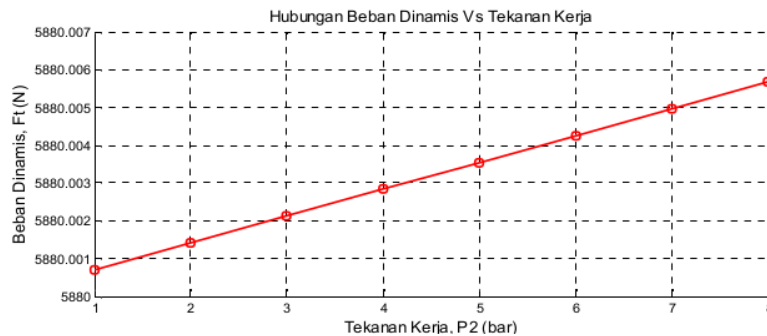
Gambar 4, Karakteristik Beban Dinamis sistem pneumatik
