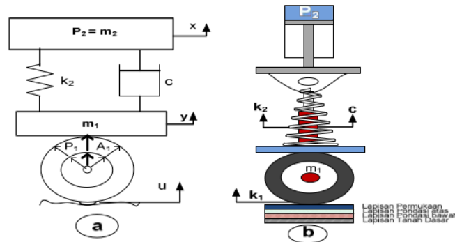
Gambar 1 (a) Model suspensi pasif (b) Unit suspensi, shock absorber, sumbu dan roda pada struktur lapisan jalan.
