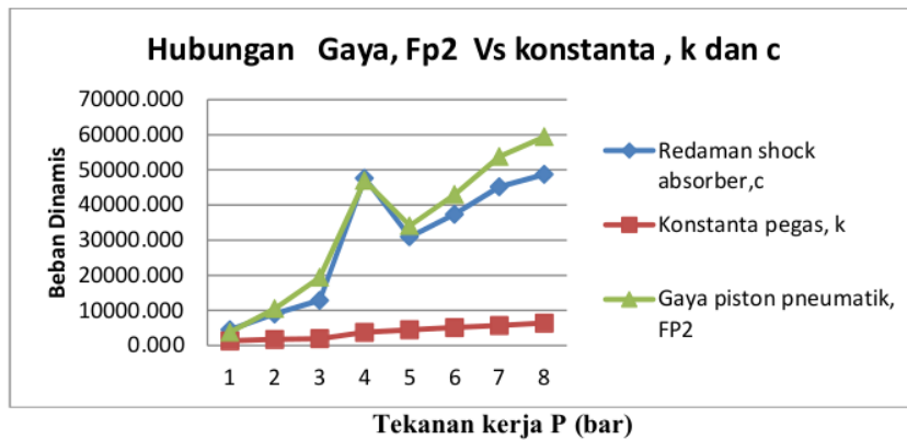
Gambar 6 Hubungan gaya piston FP2 (N) dengan peredam shock absorber dan pegas ulir
