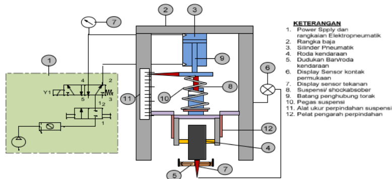
Gambar 3 Simulasi pembebanan dengan aktuator pneumatik
