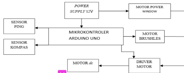
14 Gambar 2. Diagram Blok Sistem
