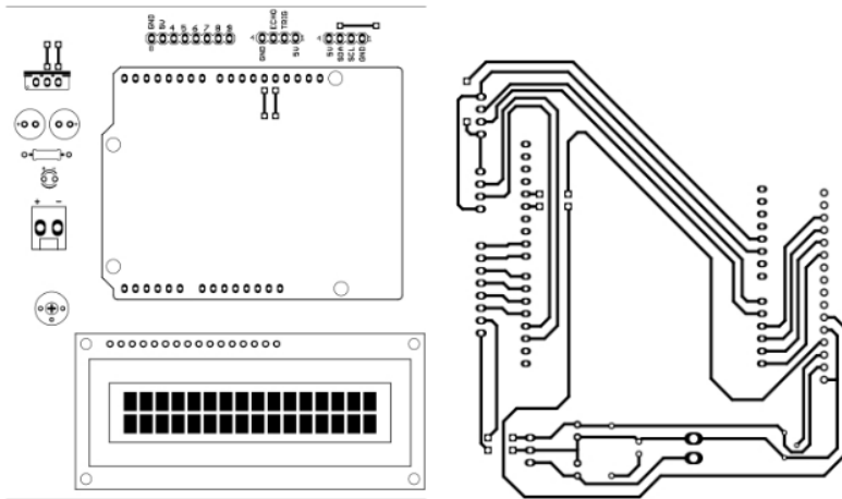
Gambar 5. Layout Skematik kontroler robot.
