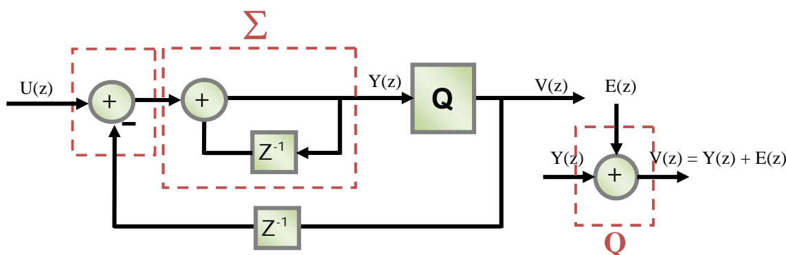
Gambar 3. Skenario skema modifikasi Delta Modulator ke Delta-Sigma Modulator dan penggunaan z-domain Delta-Sigma Modulator MOD1.
