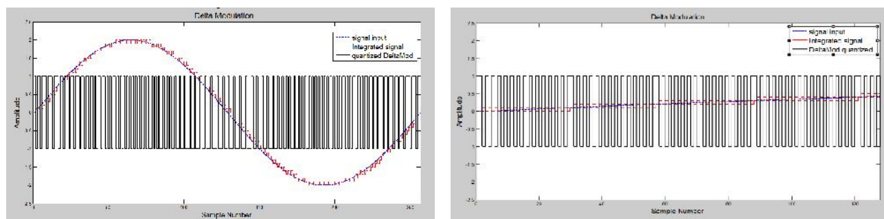
Gambar 4. Pola komparasi Delta Modulasi (kiri: pada Amplitude=2 , Bit data = 256 dan step size =0.2 dan kanan: \frac{T_{Sc}}{4} pada Amplitude=0.6 , Bit data = 1024 dan step size =0.1 ).
