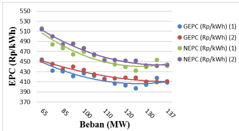
Gambar 8 Grafik Hubungan Perubahan Beban dengan Electricity Production Cost Tahun 2018
