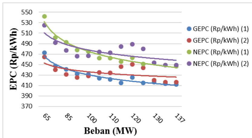
Gambar 9 Grafik Hubungan Perubahan Beban dengan Electricity Production Cost Tahun 2019
