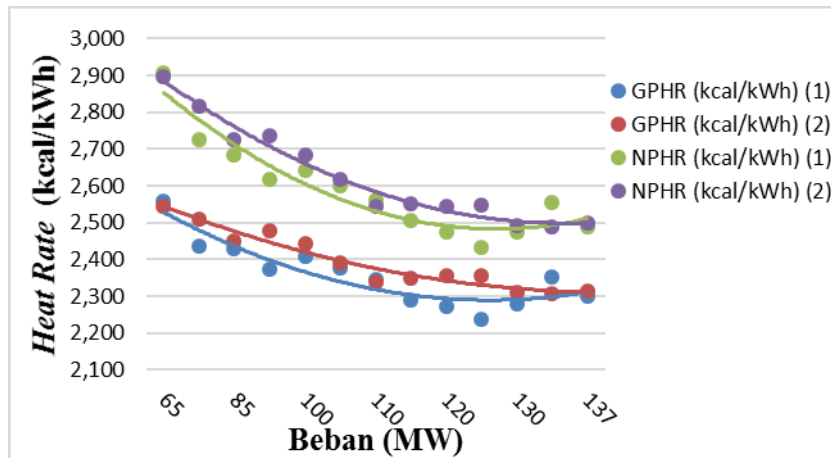
Gambar 2 Grafik Hubungan Perubahan Beban dengan Heat Rate Tahun 2018
