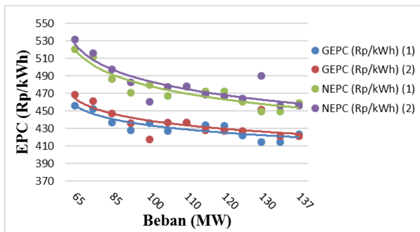
Gambar 10 Grafik Hubungan Perubahan Beban dengan Electricity Production Cost Tahun 2020
