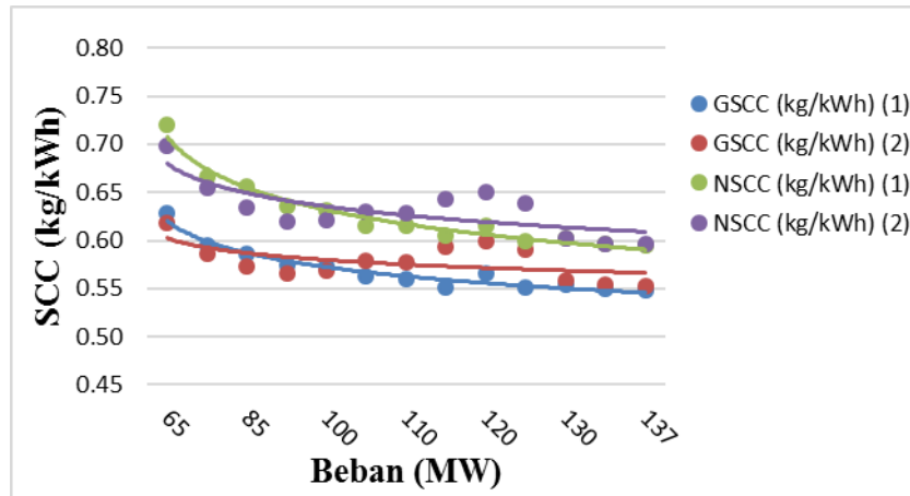
Gambar 6 Grafik Hubungan Perubahan Beban dengan Specific Coal Consumption Tahun 2019
