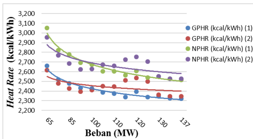
Gambar 3 Grafik Hubungan Perubahan Beban dengan Heat Rate Tahun 2019
