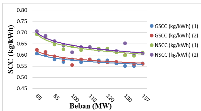
Gambar 7 Grafik Hubungan Perubahan Beban dengan Specific Coal Consumption Tahun 2020
