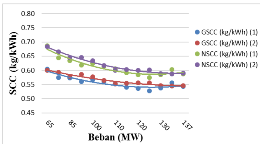
Gambar 5 Grafik Hubungan Perubahan Beban dengan Specific Coal Consumption Tahun 2018
