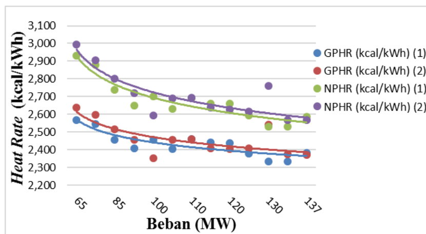
Gambar 4 Grafik Hubungan Perubahan Beban dengan Heat Rate Tahun 2020
