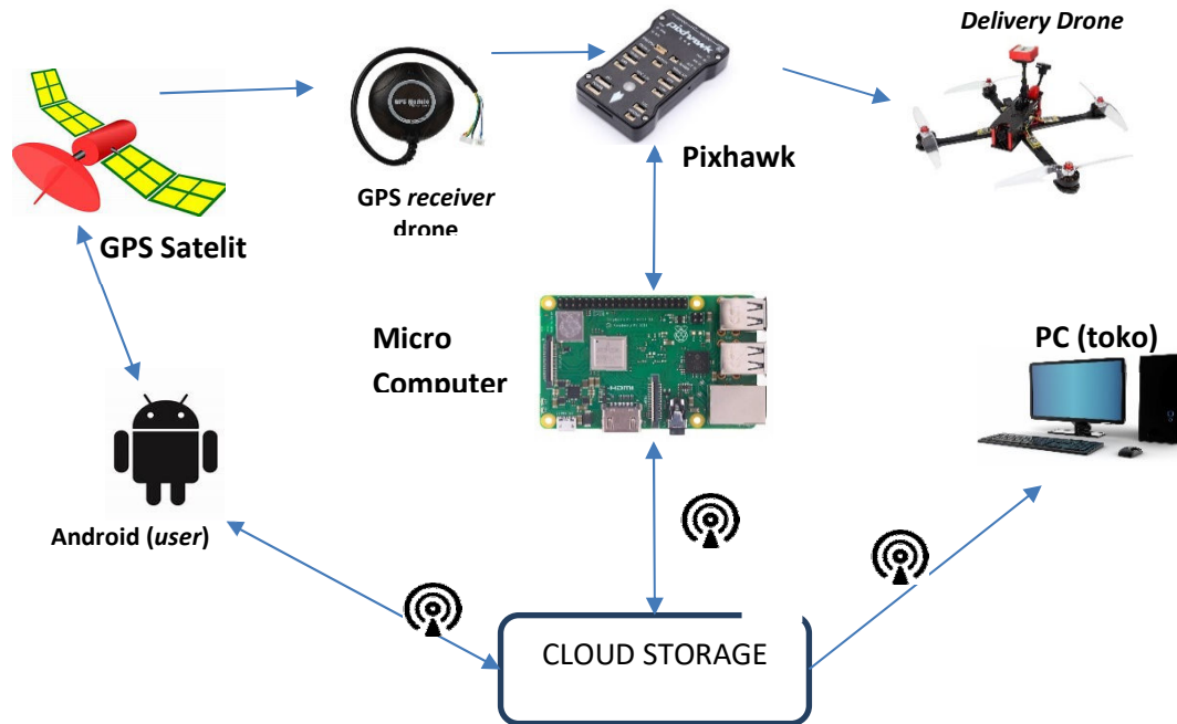
Gambar 2 Skematik diagram sistem drone
