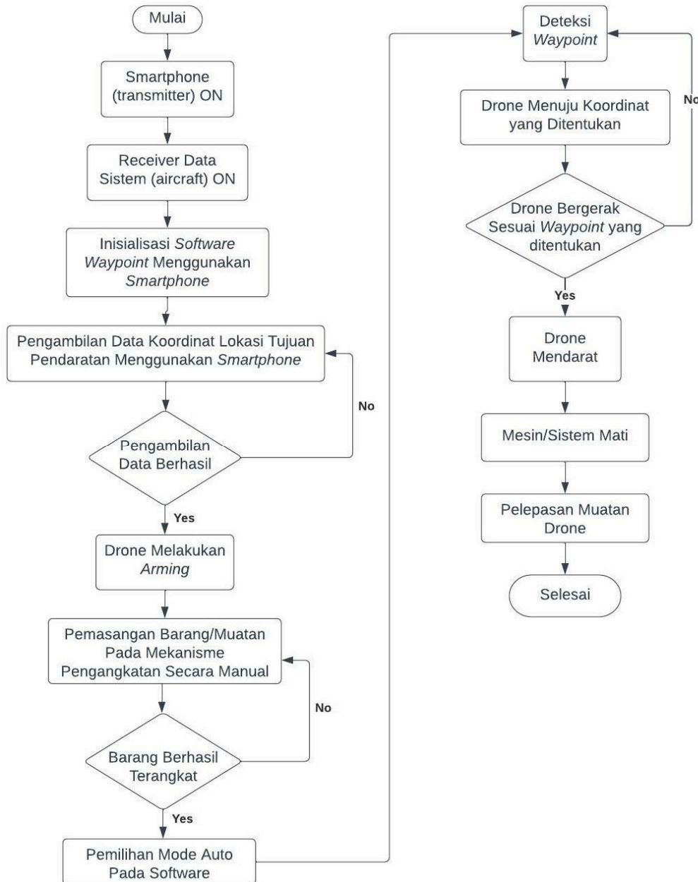
Gambar 1 Diagram alir sistem drone pengantar barang
