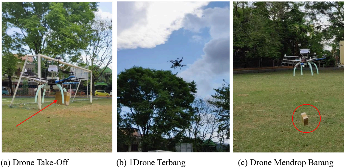
Gambar 10. Proses Pengujian Drone Terbang Membawa Barang Secara Otomatis
